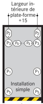
Marquage selon ISO 3864
